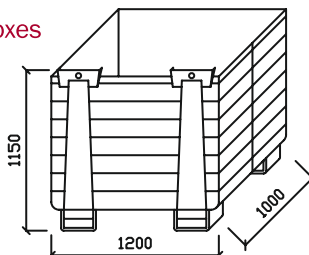
Nízkokapacitná debna Low-capacity box
